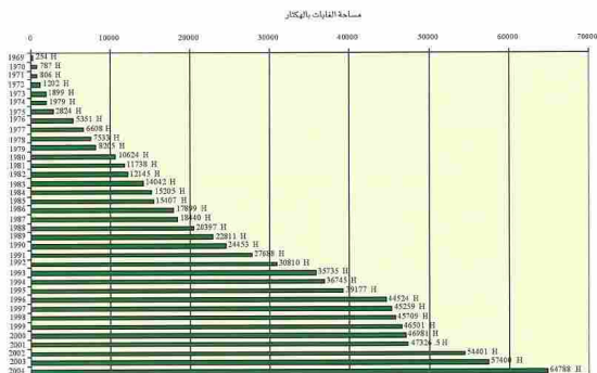
شكل ١٦. تطور الغابات (المساحة بالهكتار H) في المنطقة الشرقية من إمارة أبوظبي (٢١/٦).
