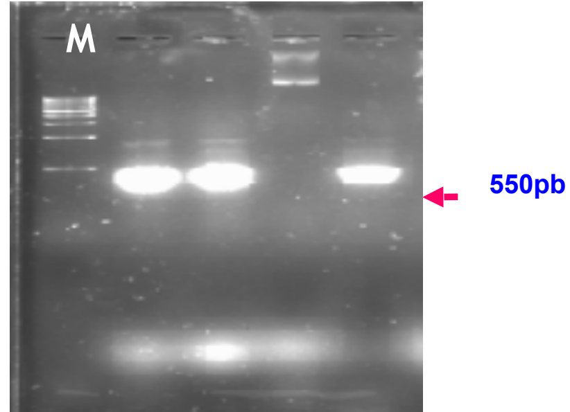
تضاعف لقطع من جين الـ SRY full fragment باستخدام تقنية الـ PCR و التي تم عمل كلونة لها في بلازميد pGEMT vector والتي ادخل بها قطع الجين المعزول لبعض اصناف النخيل (lane 2,3 and 5 for Burhi, Khalas and Sukari) توضح الصورة مقارنتها مع القياسي M DNA 1 KB. Marker
