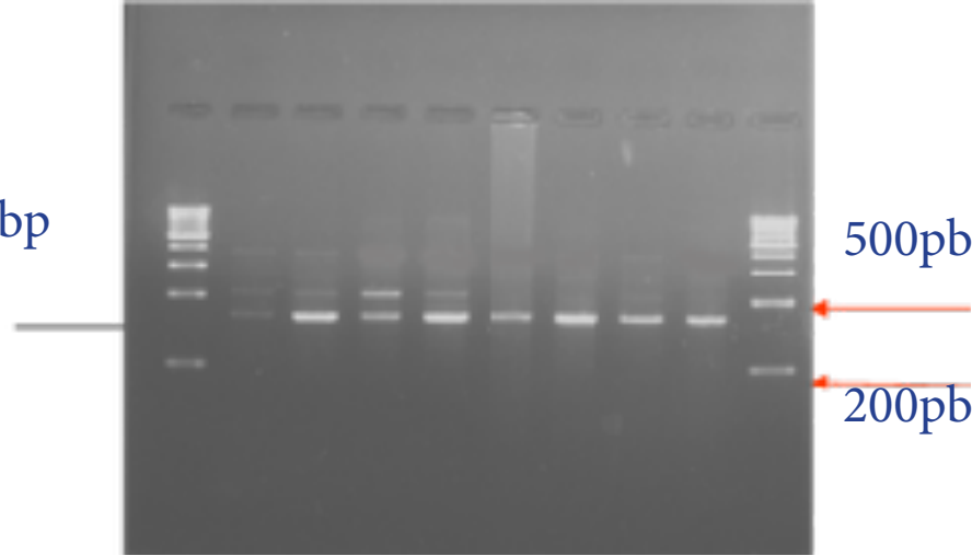
M DNA 1 KB Marker. تضاعف لقطع من جين ال SRY (387 bp) باستخدام تقنية ال PCR و التي تم عزلها من نباتات مؤنثة و توضح الصورة مقارنتها مع القياسي.
