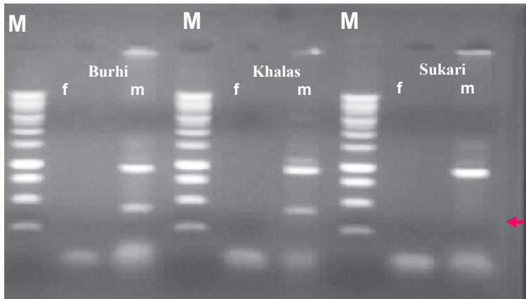
تضاعف لقطعة من جين SRY باستخدام تقنية ال PCR والتي تم عن طريقها استخدام DNA والتي تم عزلها لبعض اصناف النخيل المؤنثة f= female plantand (Burhi, Khalas and Sukari) ومقارنتها مع المذكرة والتي يرمز لها m. وتوضيح الصورة مقارنتها مع القياسي M DNA 1 KB Marker.
