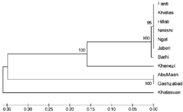
الشكل 1. الشجرة الوراثية لجين الترميز الجيني matK باستخدام UPGMA
