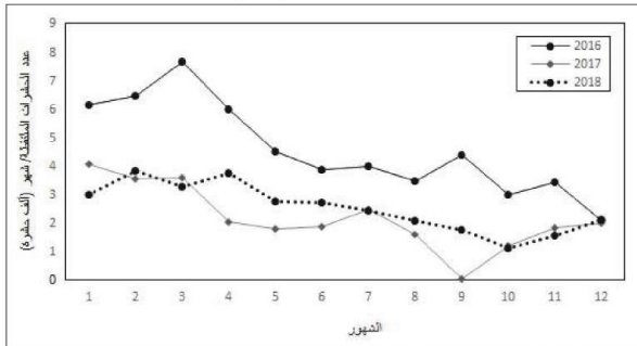
شكل رقم (10) الأعداد الشهرية الملتقطة للطور الكامل لحشرة سوسة النخيل الحمراء من المصائد الفرمونية التجميعة خلال الفترة 2016-2018
