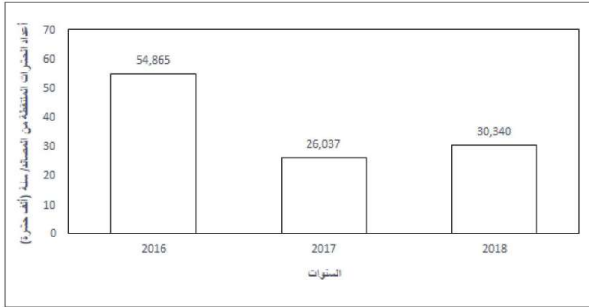
شكل رقم (11) الأعداد الكلية الملتقطة للطور الكامل لحشرة سوسة النخيل الحمراء من المصائد الفرمونية التجميعية خلال الفترة 2018-2016
